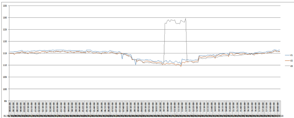
Figura 2 Valores nominales de diferencia de potencial en las 3 fases. Fuente Elaboración propia.
