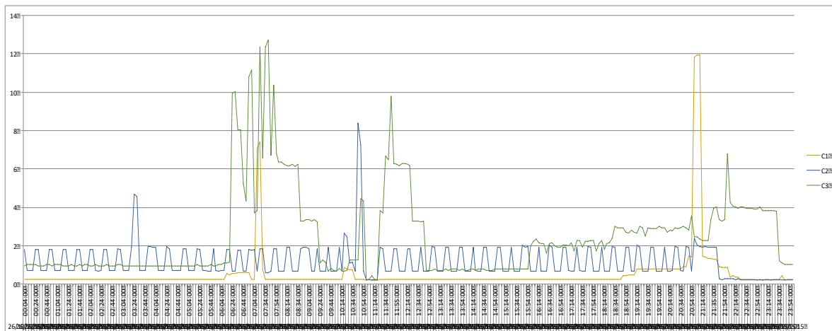
Figura 4.- Pruebas de carga en las fases. Fuente: Elaboración propia.
